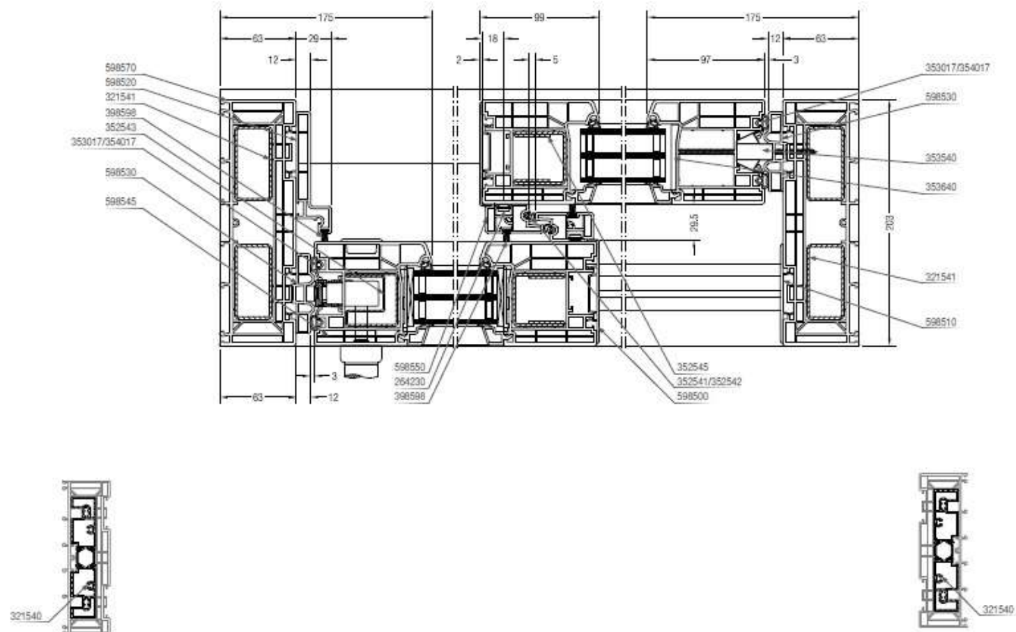
Sezione nodo scorevole alzante ( vista da sopra )
